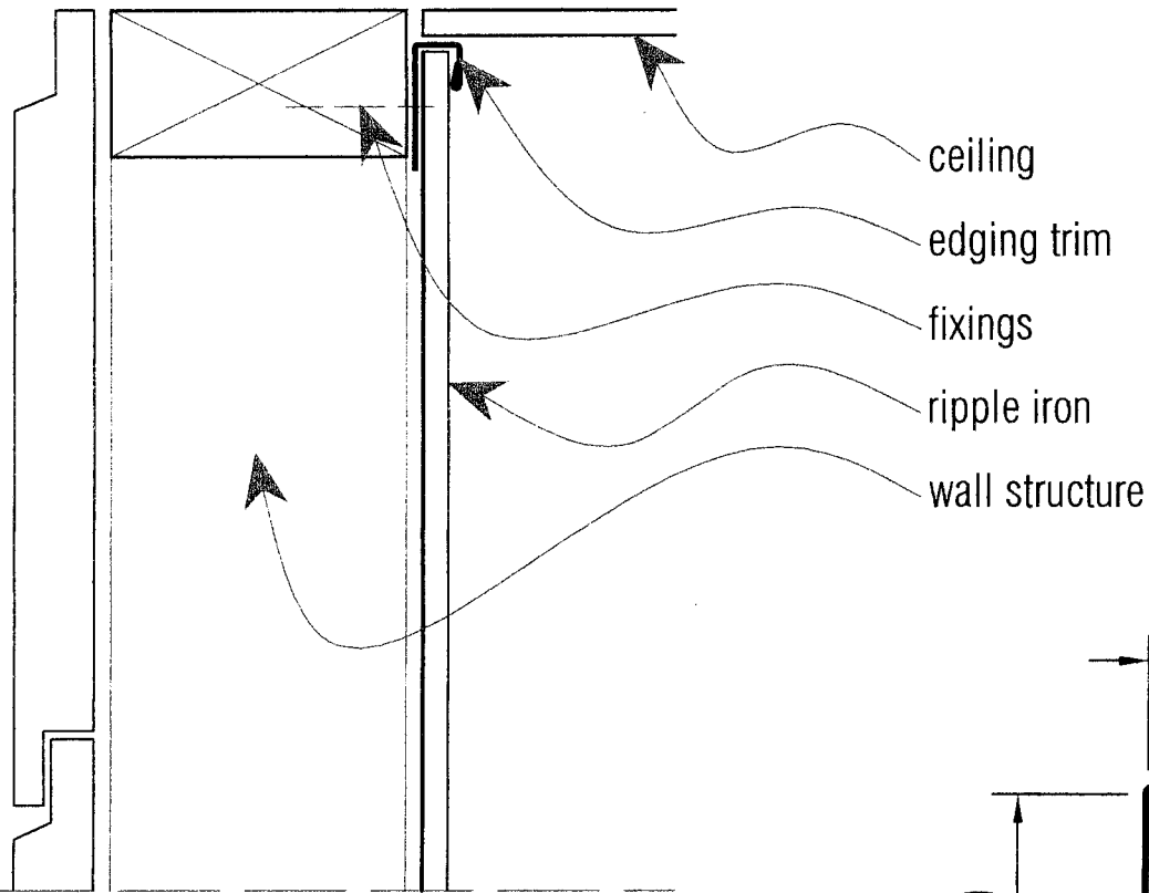
SECTION OF EDGING TRIM scale: 1 : 2 @ A4
