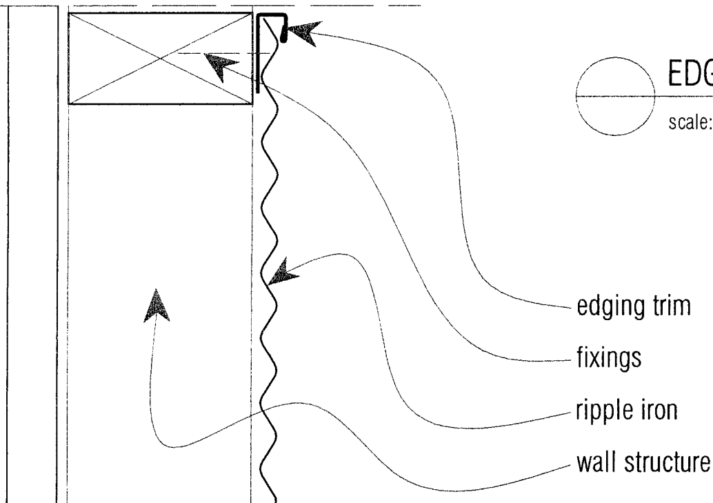
PLAN OF EDGING TRIM scale: 1 : 2 @ A4
