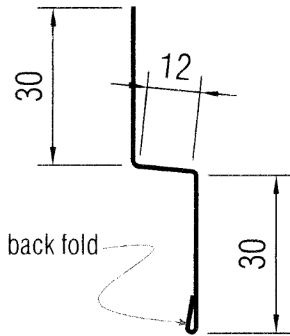
Z - FLASHING scale: 1 : 1 @ A4
